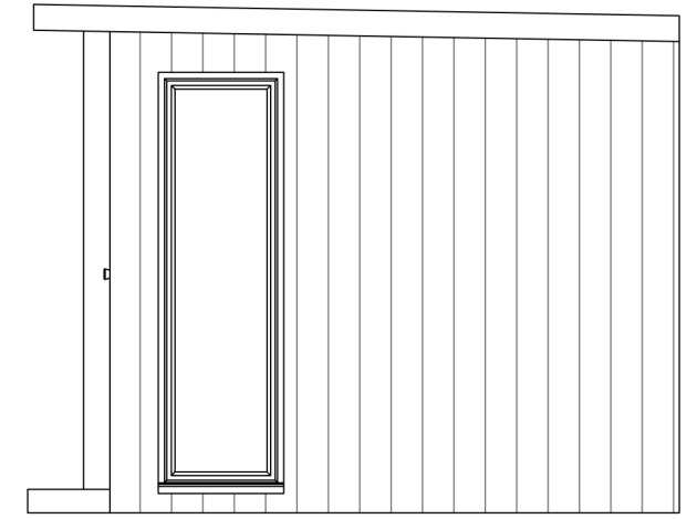
5 Right Elevation 1 : 40
